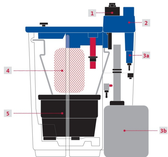
Funcionamiento del ÖWAMAT®
