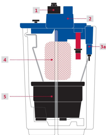
Funcionamiento del QWIK-PURE®
